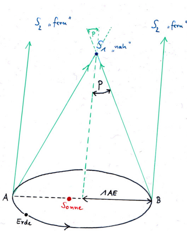
Die jährliche Parallaxe p eines Sterns
